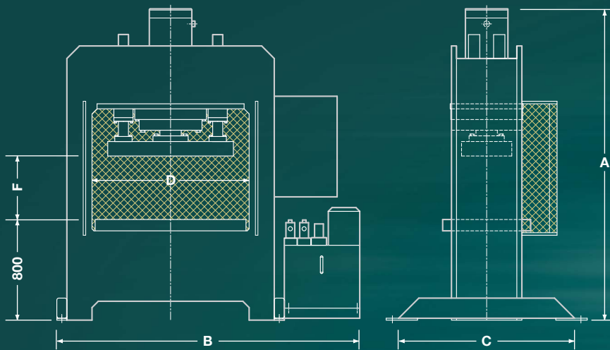
Premilamiera, Serre-tôle, Blank-holder, Blechhalter, Cojín
